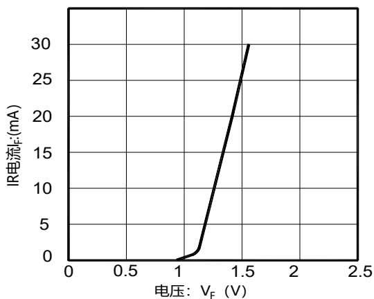
图5 IR电流与电压
